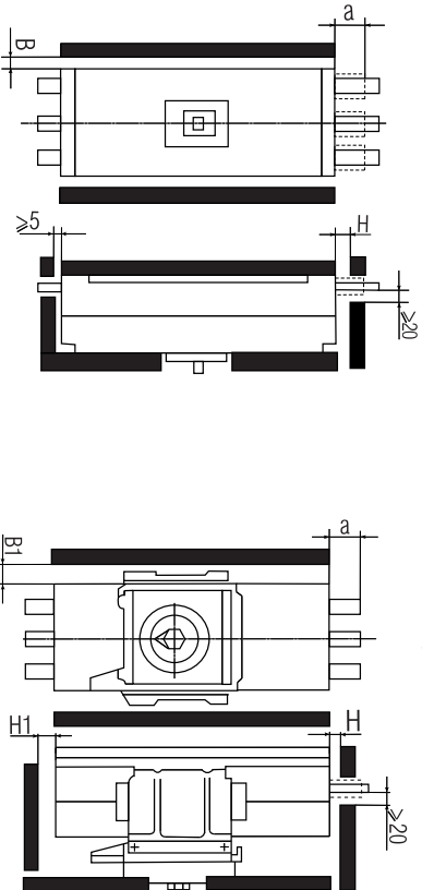
Выключатель выдвижного исполнения с ручным дистанционным или электромагнитным приводом
