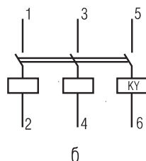
Рисунок 28 - Схема электрическая принципиальная выключателя А3792Б
