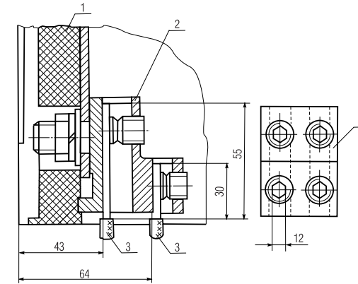
1 - выключатель; 2 - зажим; 3 - присоединяемая шина. Рисунок 8 - Зажим винтовой для переднего присоединения к главной цепи выключателя шины, а также провода или кабеля с кабельным наконечником (кабельный наконечник на рисунке не показан).
