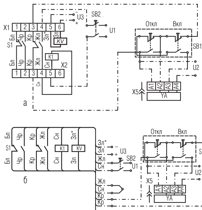
Рисунок 32 - Схема электрическая соединений дополнительных свободных контактов выключателей
