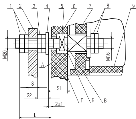
Рисунок 10 - Зажим для переднего присоединения с переходной шиной.
