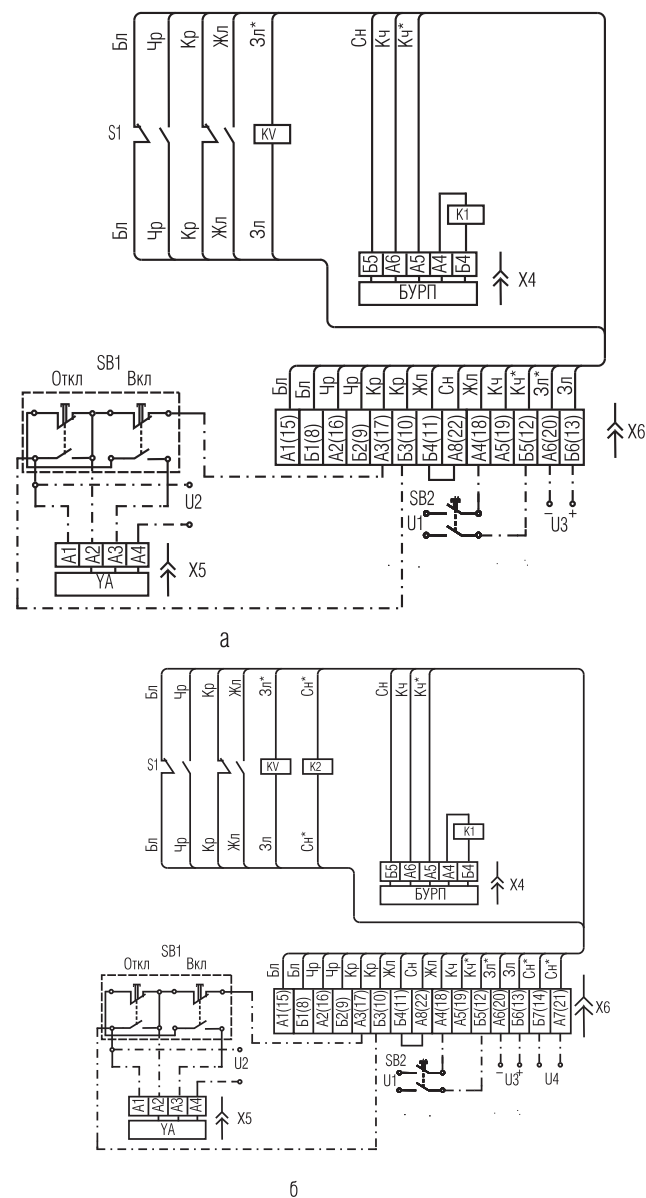
а - выключателей А3793 Б и А3794Б ; б - выключателей А3793Б, А3794Б, А3793С и А3794С. Рисунок 31 - Схема электрическая соединений дополнительных сборочных единиц выключателей выдвижного исполнения
