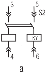
Рисунок 25 - Схема электрическая принципиальная выключателя А3797С
