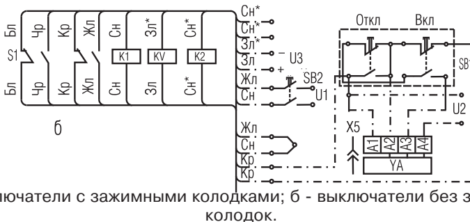
Рисунок 35 - Схема электрическая соединений дополнительных сборочных единиц выключателей стационарного исполнения А3791Б, А3792Б
