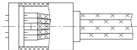
Рисунок 42- Вилка соединительная.
