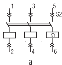
Рисунок 26 - Схема электрическая принципиальная выключателя А3798С
