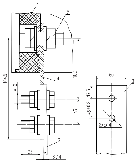
Рисунок 10 - Зажим для переднего присоединения с переходной шиной.
