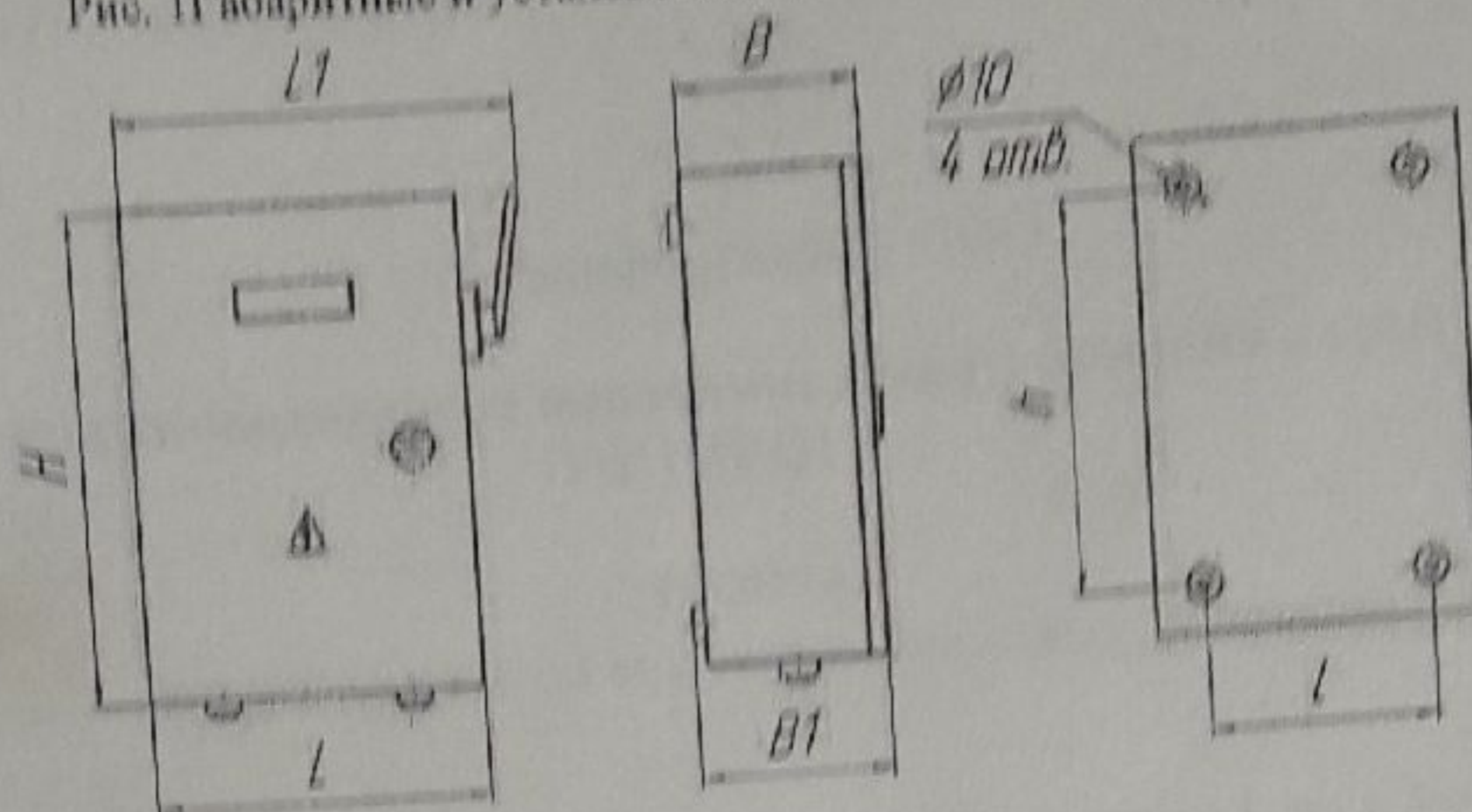
Рис. 1 Габаритные и установочные размеры ящиков ЯРП-1/2/4
